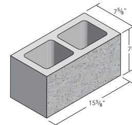
8x8x16 Standard
