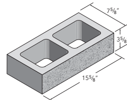
8x4x16 Standard
