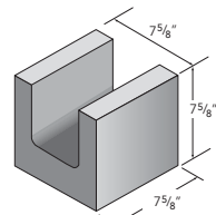
8x8x8 Lintel
