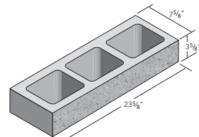
8x4x24 Standard
