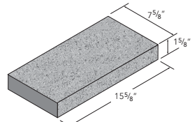
8x2x16 Cap
