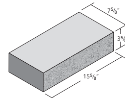
8x4x16 Solid
