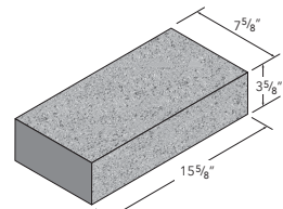
8x4x16 Cap
