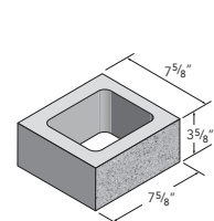
8x4x8 Standard
